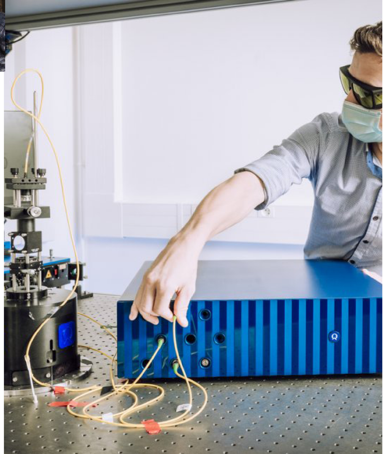
La fibre optique tenue en main par l'expérimentateur véhicule des photons uniques (qubits photoniques) issus d'une source semi-conductrice (boîte quantique, non visible) placée dans le cryostat noir à gauche de la photo. Ces photons uniques sont collectés par le biais d'un microscope confocal positionné au-dessus de la chambre du cryostat. Puis les photons uniques sont filtrés en séparant le laser qui a servi pour l'excitation optique de la source. Cette étape est réalisée dans la boîte bleue baptisée QFiber qui sert d'interface entre le laser d'excitation, la source de photons dans le cryostat et le reste de l'expérience. La start-up Quandela, fondée en 2017 par Valérian Giesz, Niccolò Somaschi et Pascale Senellart (directrice de recherche CNRS), travaille sur ces qubits photoniques. Cette approche permet une exploitation simultanée de dizaines de qubits. Le qubit est l'unité de stockage de l'information qui indique la force de calcul des ordinateurs quantiques. La start-up fabrique des sources à base de boîtes quantiques d'une centaine d'atomes, qui sont miniaturisées et stabilisées.
